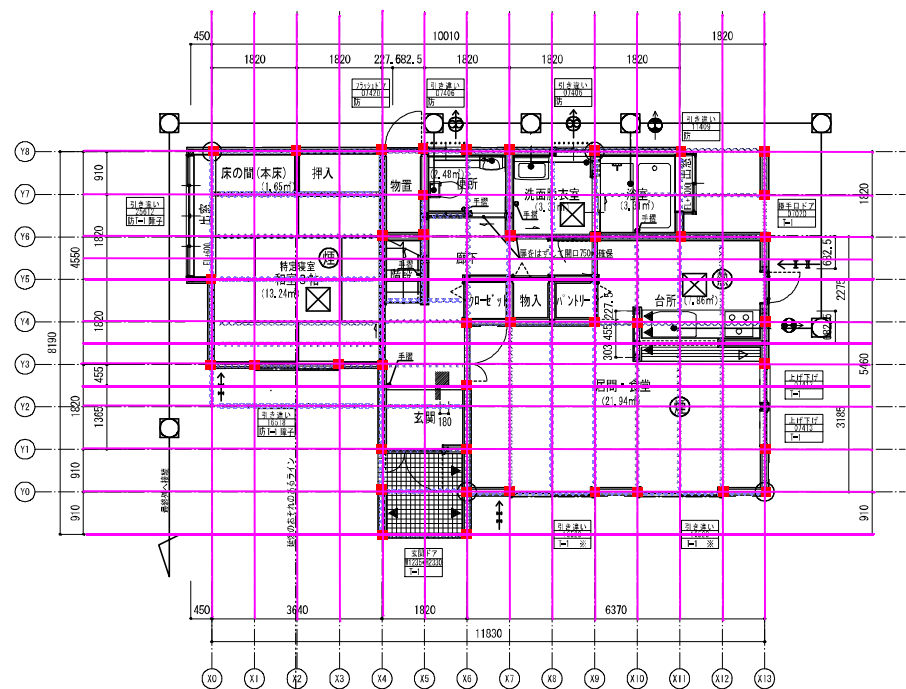
1階平面図 1/100
