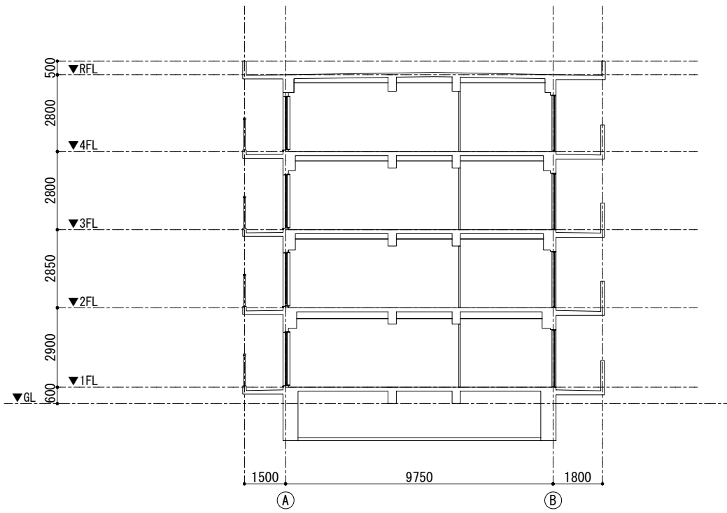
断面图
