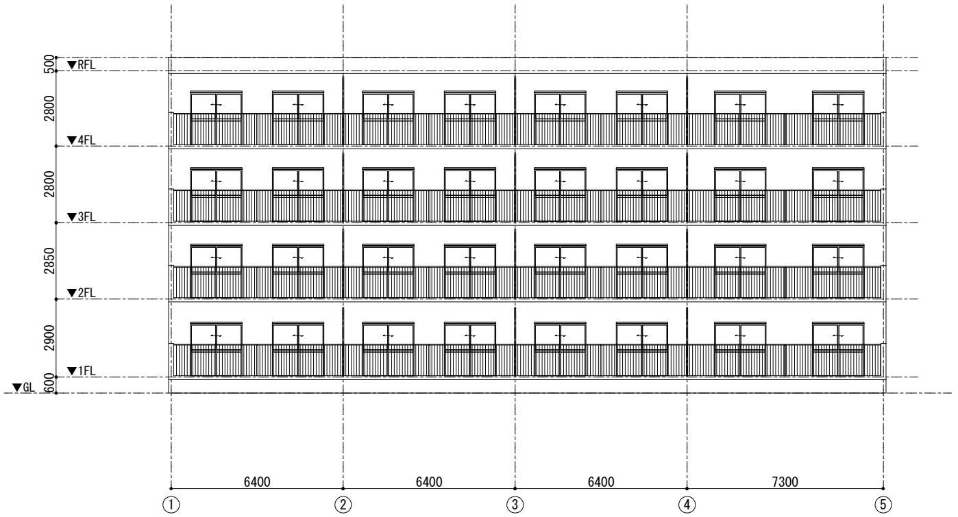
立面图
