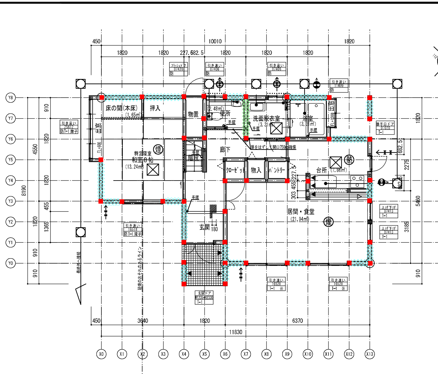
1階平面図 1/100
