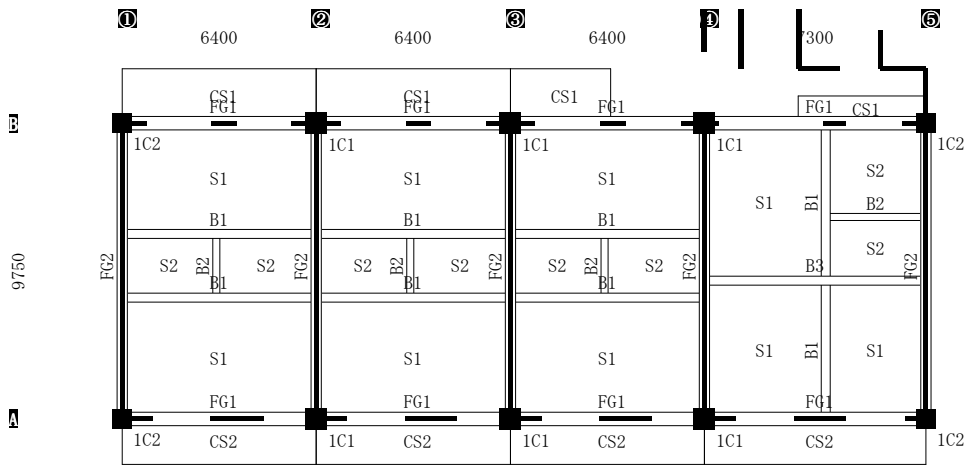
1F 階梁伏図
