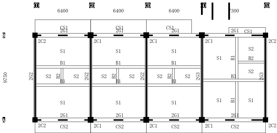
2F 階梁伏図
