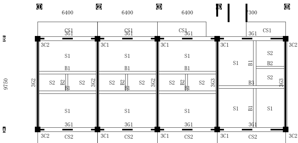
3F 階梁伏図
