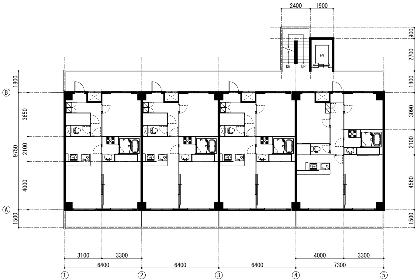
2 ~ 4 階平面図
