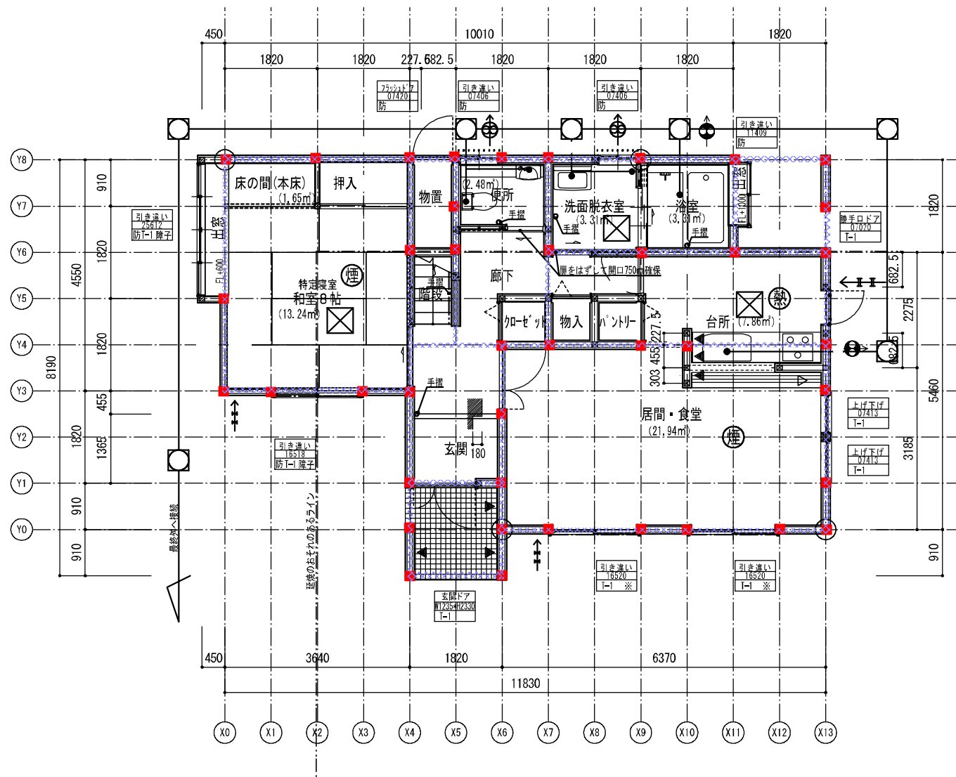
1階平面図 1/100
