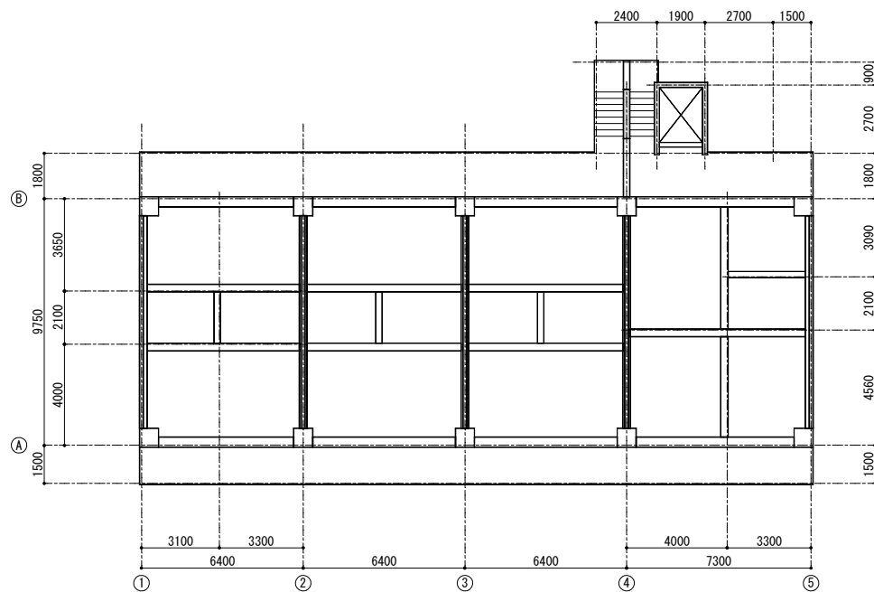
3、4階伏図
