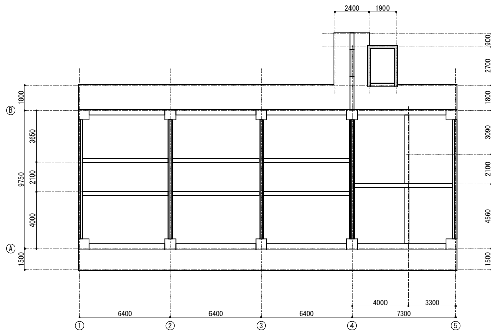
R階伏図
