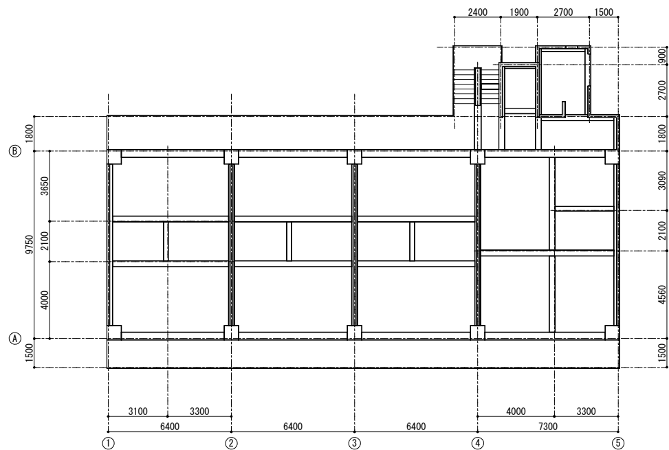
1階伏図
