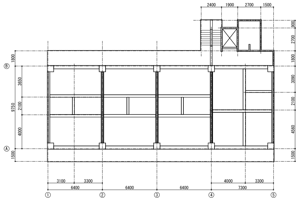
2階伏図
