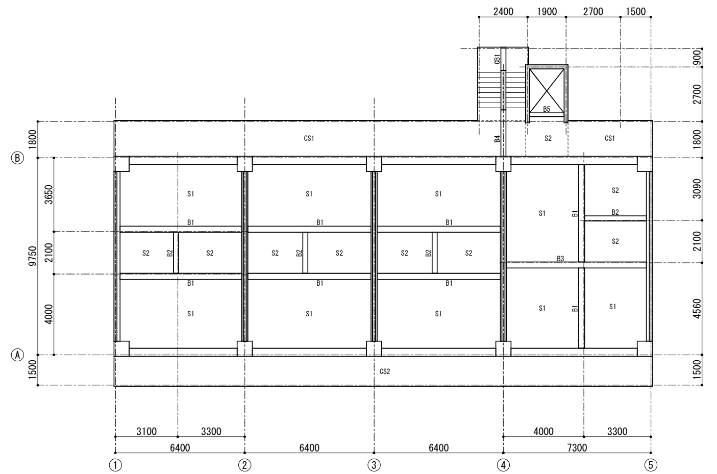
3、4階伏図
