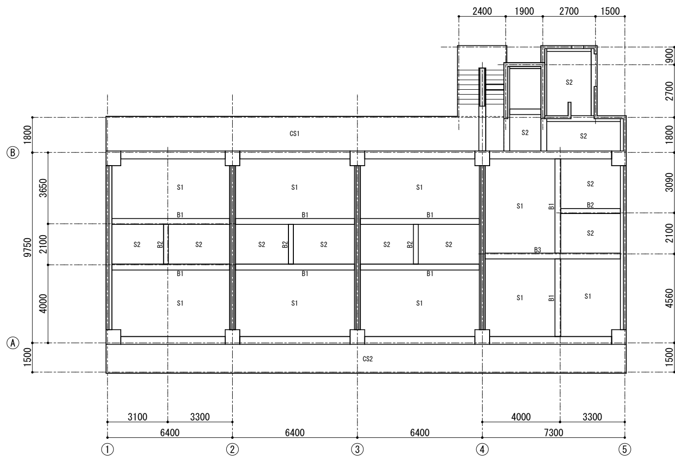
1階伏図
