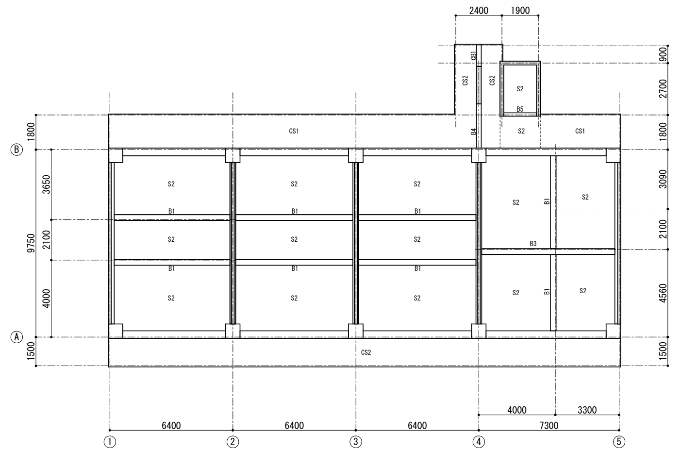
R階伏図
