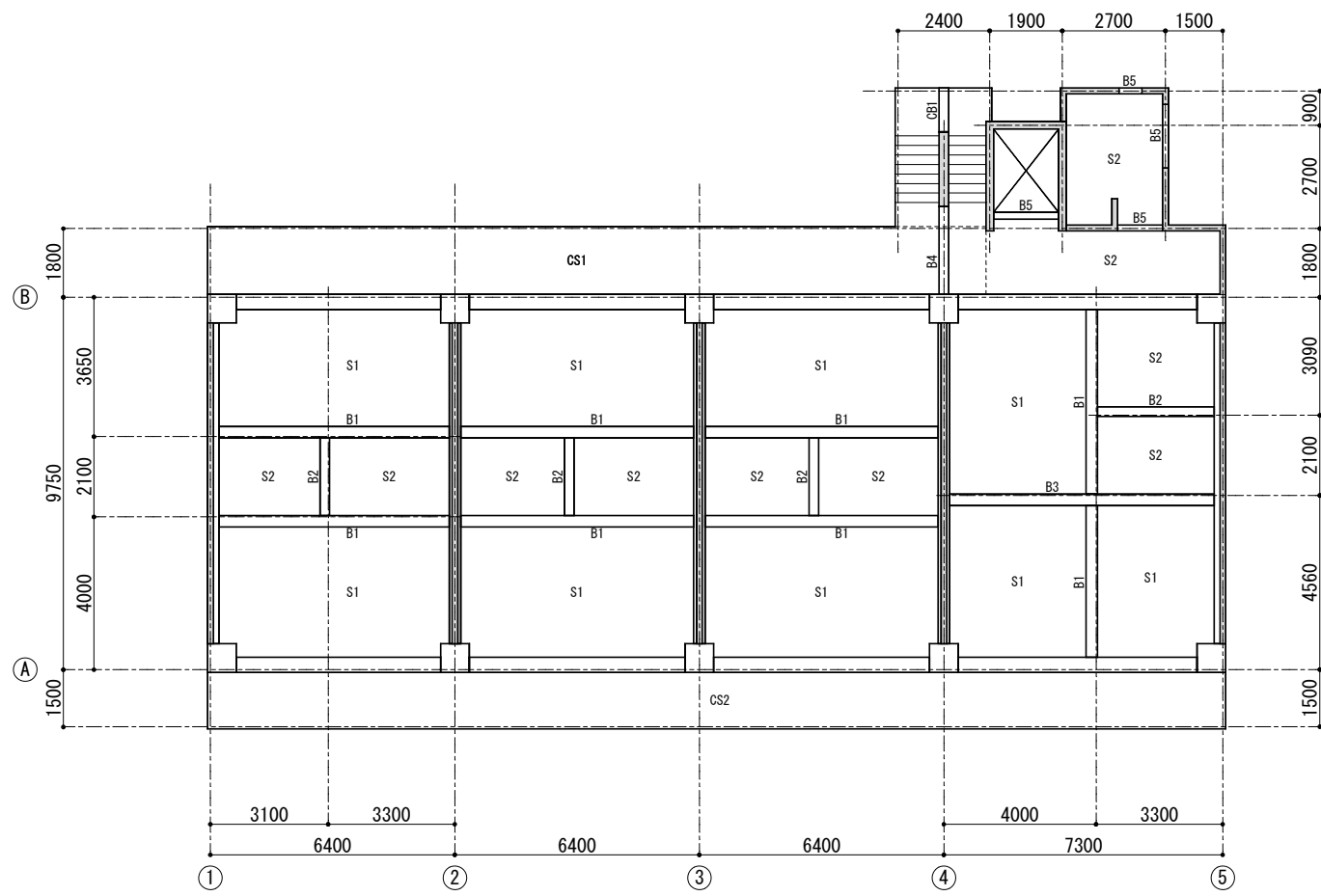
2階伏図
